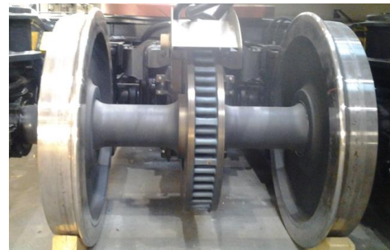
Achse und Monoblockrad
