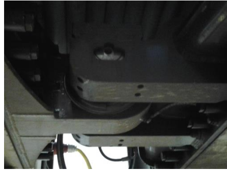
Sekundärfeder -> (Luftfeder inkl. Schichtfeder)
