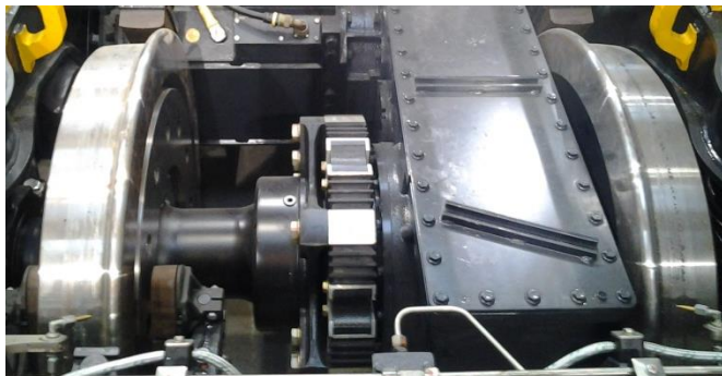
Achse und Monoblockrad
